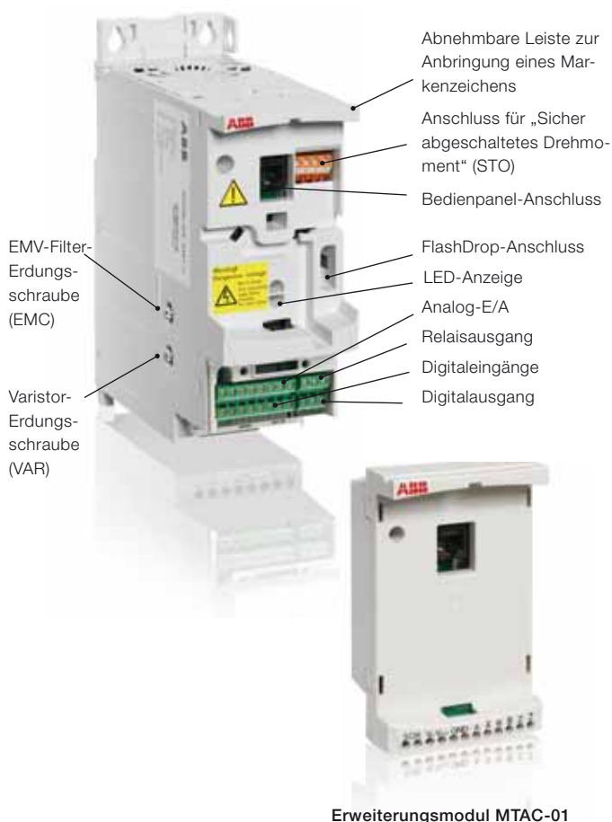
Erweiterungsmodule MTAC-01
